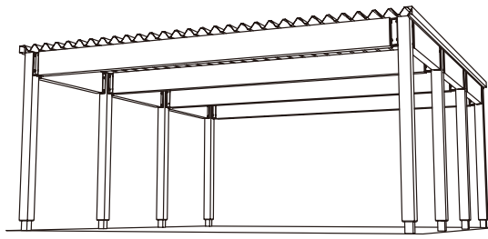
幅 5.7m 奥行 6m 開口高 2.3m
