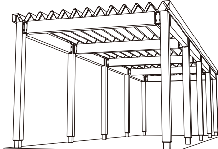
幅 3m 奥行 10.8m 開口高 2.3m
