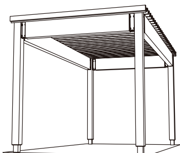
幅 2.5m 奥行 5m 開口高 2.3m
