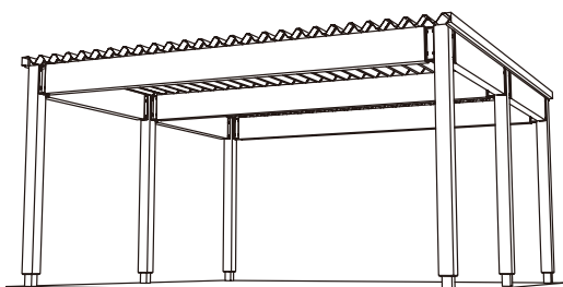
幅 5.1m 奥行 5m 開口高 2.3m
